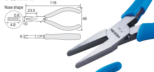
P-34 MINIATURE FLAT NOSE PLIERS 小型扁嘴钳
