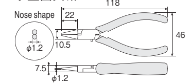
P-39 MINIATURE ROUND NOSE PLIERS 小型圆夹钳
