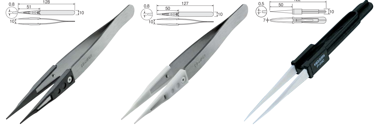
P-646-D ESD CERAMIC TIP TWEEZERS 防静电陶瓷镊子
