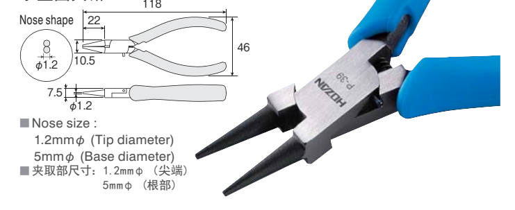
P-39 MINIATURE ROUND NOSE PLIERS 小型圆夹钳
