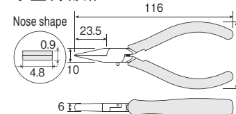
P-34 MINIATURE FLAT NOSE PLIERS 小型扁嘴钳
