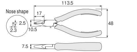
P-39 MINIATURE ROUND NOSE PLIERS 小型圆夹钳
